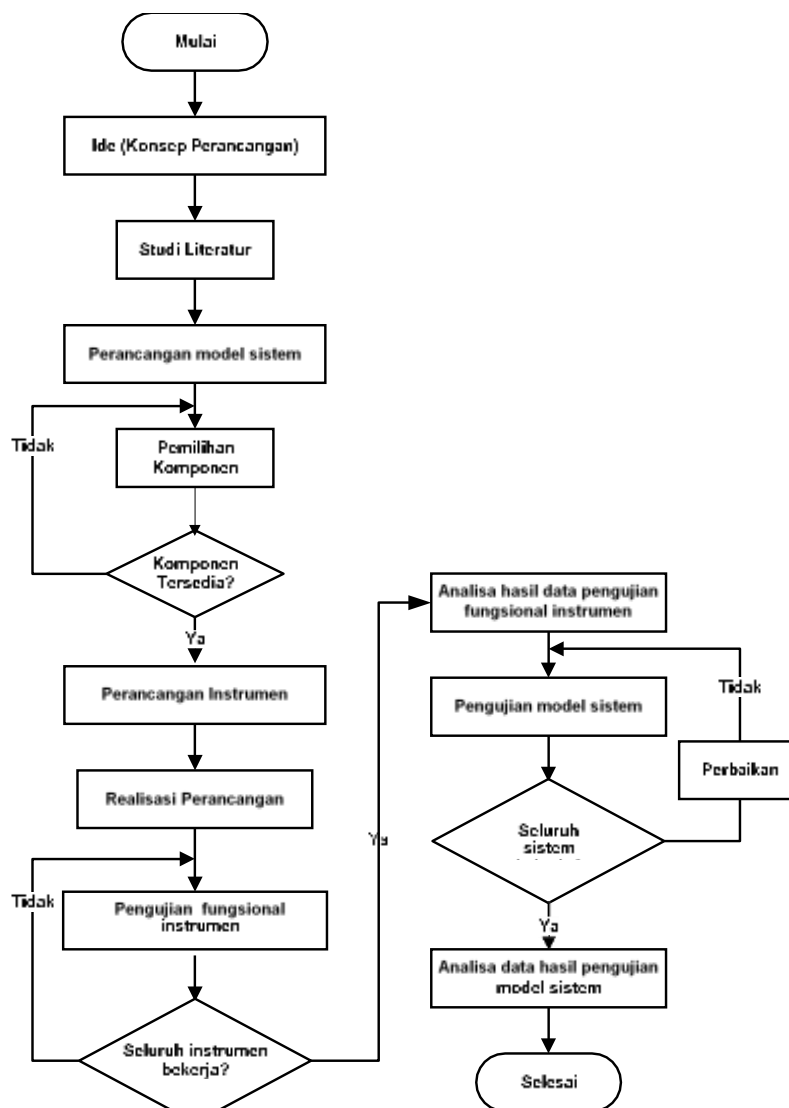
Gambar 2. Langkah kerja sistem monitoring lampu lalu-lintas
