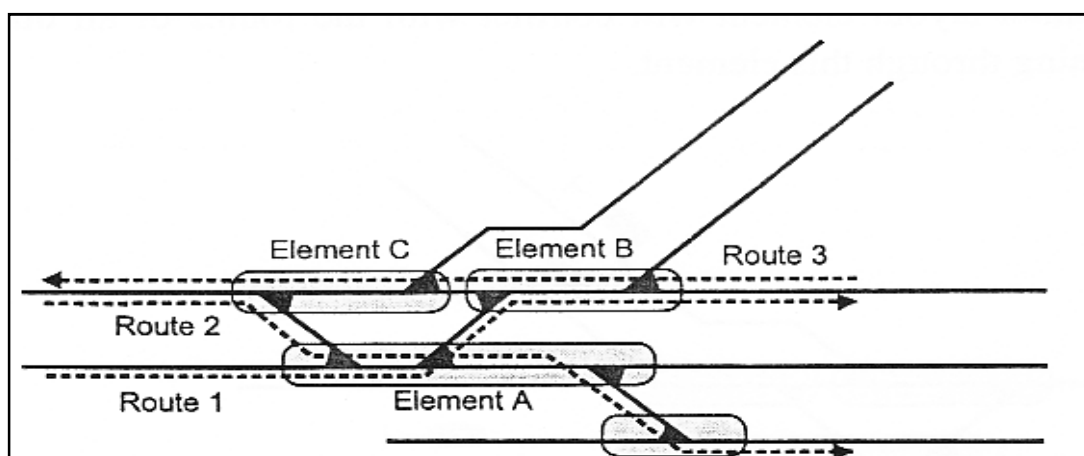
Gambar 4 Contoh Hubungan Saling Keterkaitan diantara 3 Rute (Pachl, 2004)
