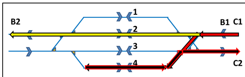
Gambar 10 Rute B vs Rute C (Divergen)
