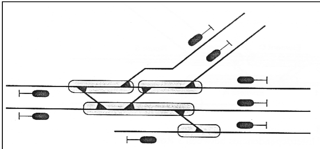
Gambar3 Pembagian sistem Interlocking menjadi beberapa kelompok wesel(Pachl, 2004)
